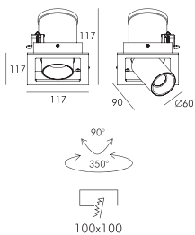
GL7117-1/1 x 12W
