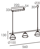
HL77026/3x6W
