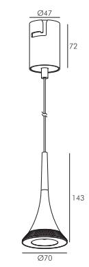
SL74135-MZ09/7W
