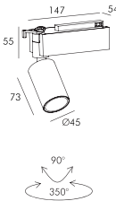
TL2022/7W
