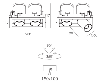
GL7117-2/2 x 12W
