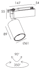
TL2023/12W
